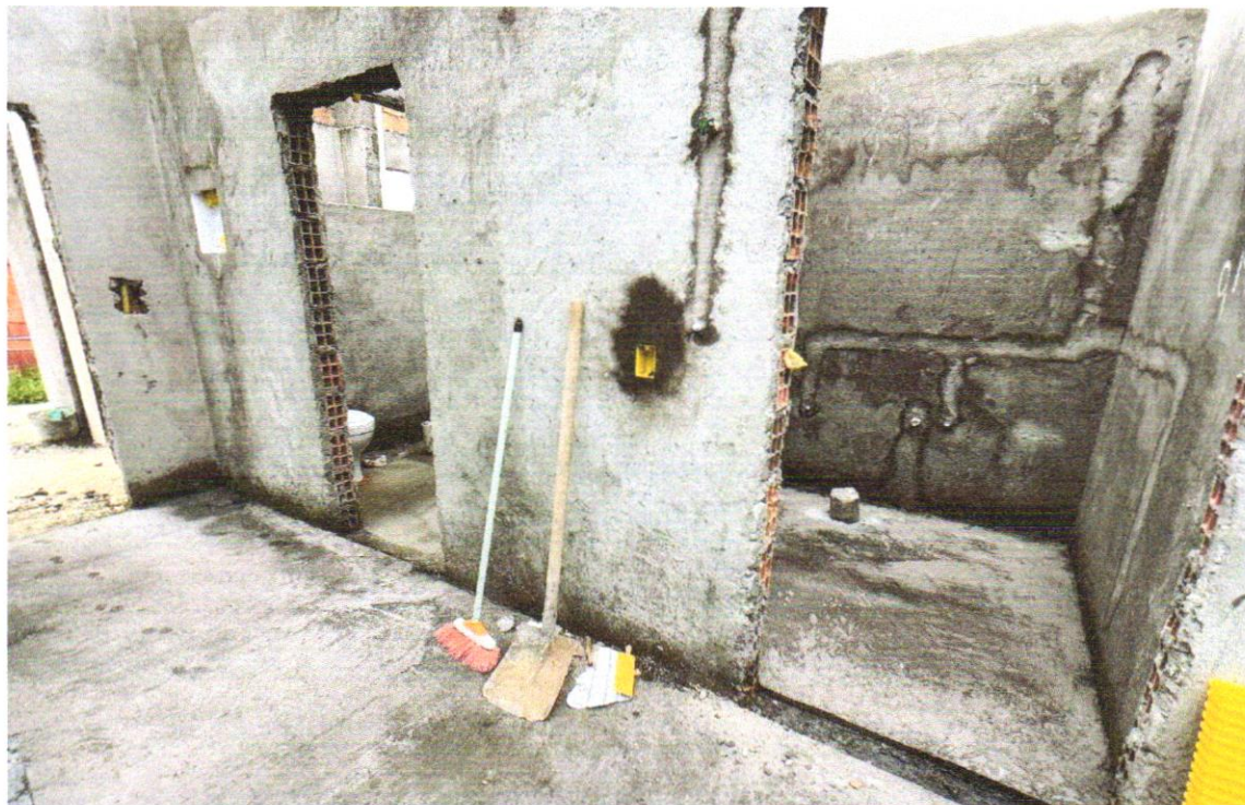
FOTO 36 – Caixa de passagem PVC 4x2"
