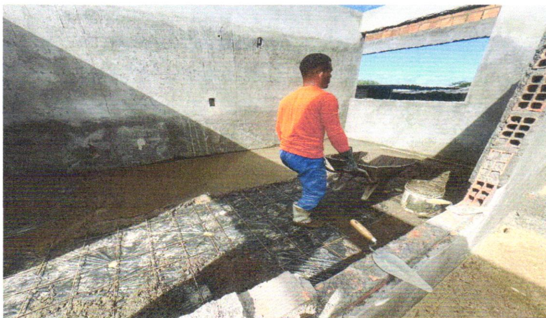
FOTO 39 – Contrapiso de concreto não-estrutural, espessura 3cm e preparo mecânico
